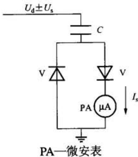
图3 用电容器和整流电路测量纹波
