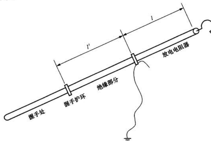
图 6 放电棒的尺寸
