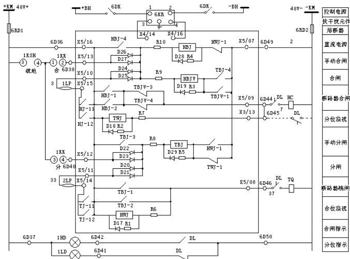
10KV 电容器保护装置原理图
