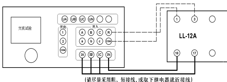
LL-12A 过电流继电器的接线图。
