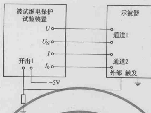
图 12 合闸相位角试验接线图
