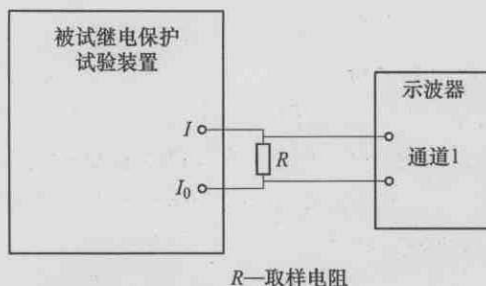
图 2 交流电流响应速度测量接线图
