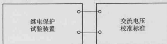
图 4 交流电压的幅值误差校准接线示意图
