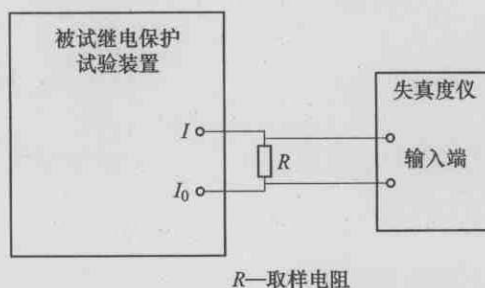
图 3 交流电流总谐波畸变率测量接线图
