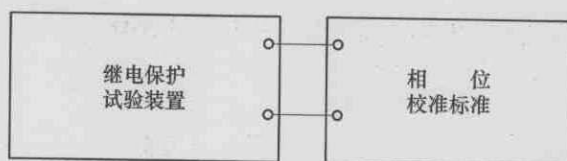
图 11 相位校准接线示意图
