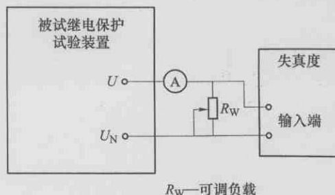
图 6 交流电压总谐波畸变率测量接线图
