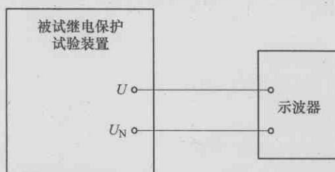
图 5 交流电压响应速度测量接线图
