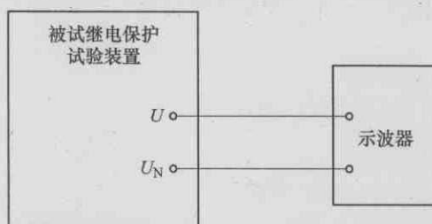
图 5 交流电压响应速度测量接线图
