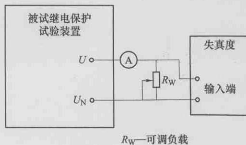
图 6 交流电压总谐波畸变率测量接线图
