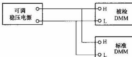
图 3 直接比较法接线
