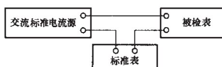
图 10 交流标准电流源法接线
