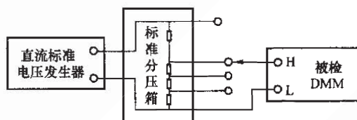
图 2 直流标准电压发生器法接线（二）
