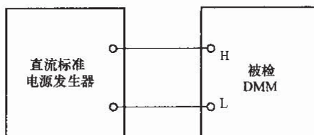
图 1 直流标准电压发生器法接线（一）
