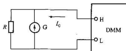
图 16 零电流测试
