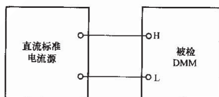
图 5 直流标准电流源法接线
