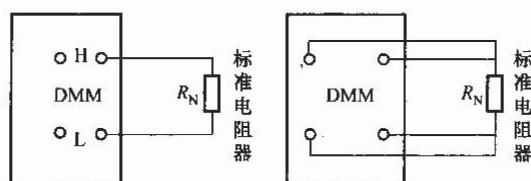
图 13 标准电阻器法
