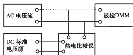
图 8 热电比较法接线
