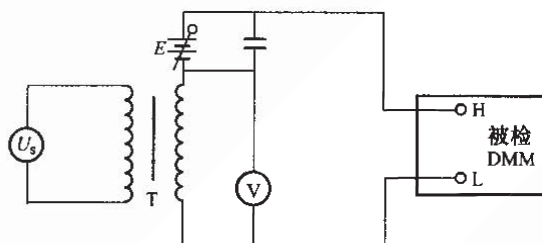
图 18 SMR (NMR) 的测试电路
