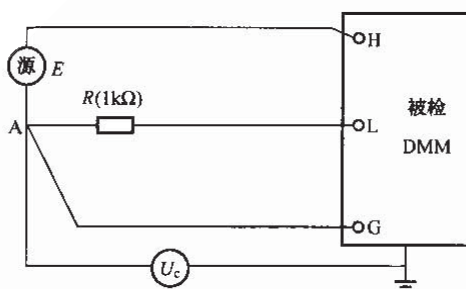
图 19 共模干扰抑制比 (CMR) 的测试
