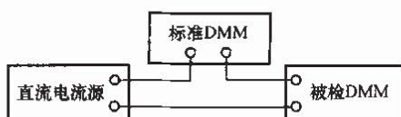
图6 直接比较法检定接线
