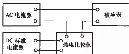
图 12 热电比较法
