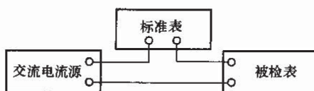
图 11 比较法检定接线
