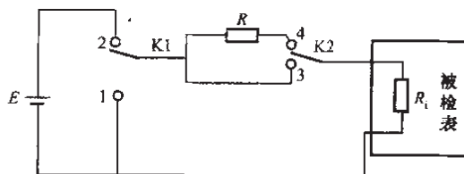
图 15 直流电压部分的输入电阻测试
