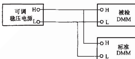
图7 比较法检定接线
