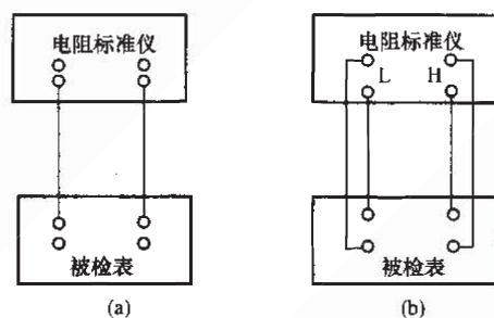
图 14 电阻校准仪法接线
