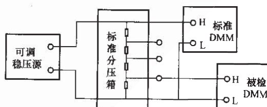
图 4 标准分压箱扩展量程接线
