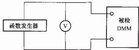
图 20 波峰因数的测试
