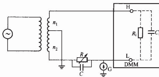
图 17 交流电压输入阻抗测试
