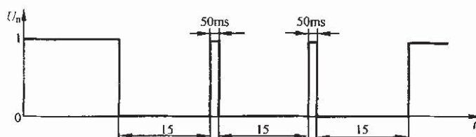
图 A.1 电压中断为 \Delta U = 100\% , 1s
