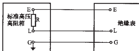
R—标准电阻; E—接地端子; L—测量线路端子; G—屏蔽端子
